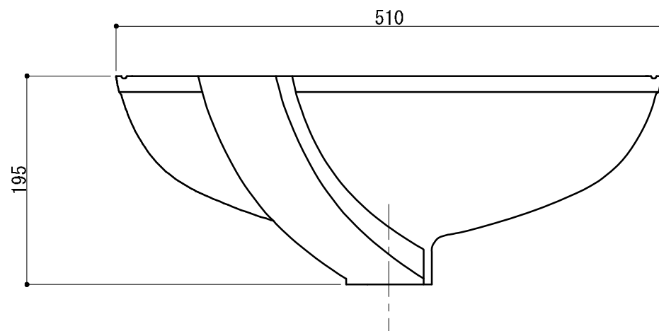
正面図
