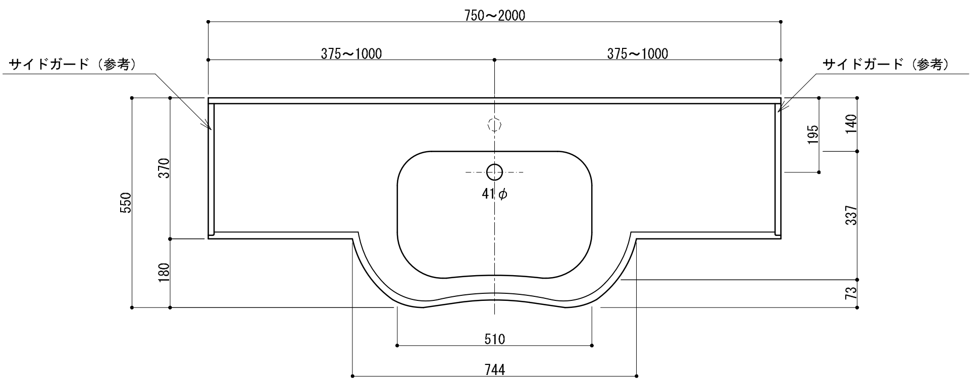
平面図
