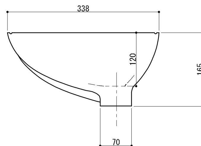
側面図
