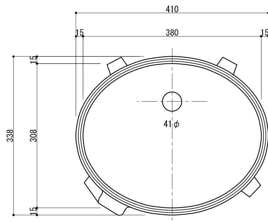
平面図
