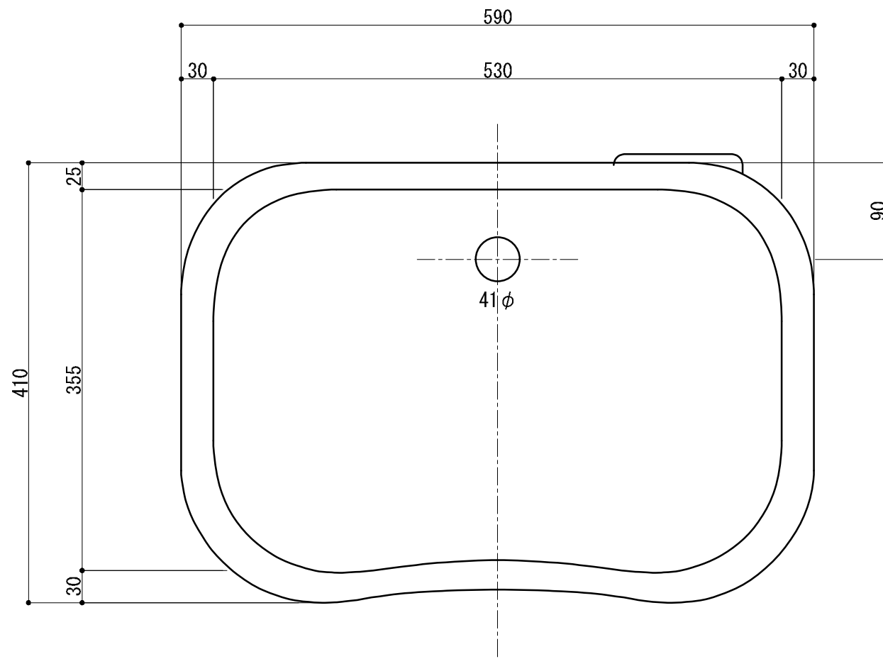
平面図
