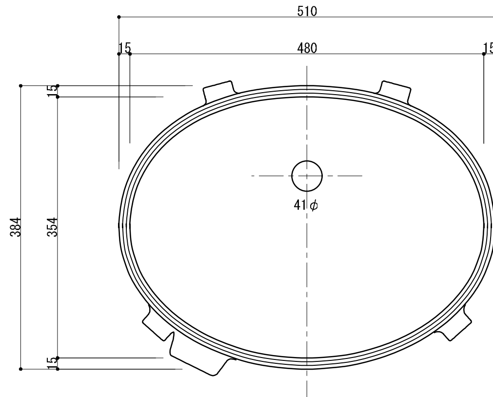
平面図
