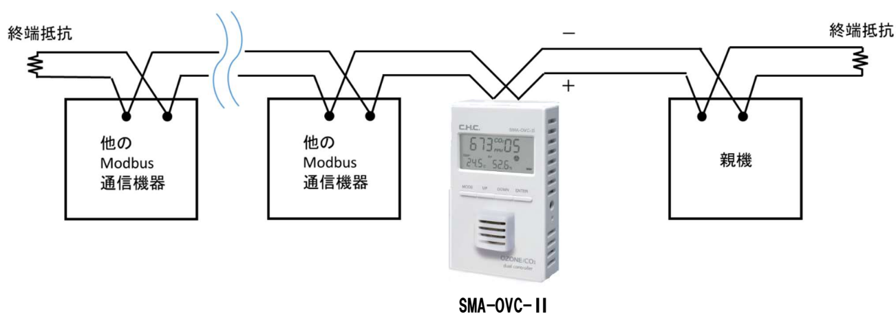
図2：Modbus 通信機器 接続方法
