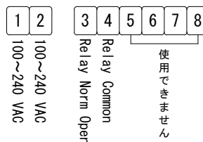
配線端子
